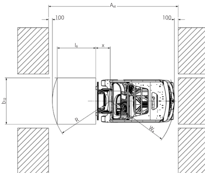
Bovenaanzicht 4 wielen
