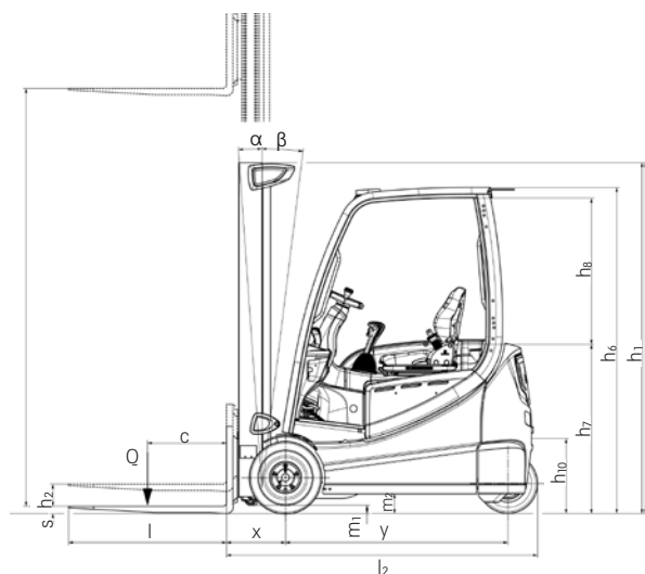
Zijaanzicht 3 wielen
