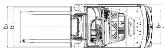
Bovenaanzicht 4 wielen
