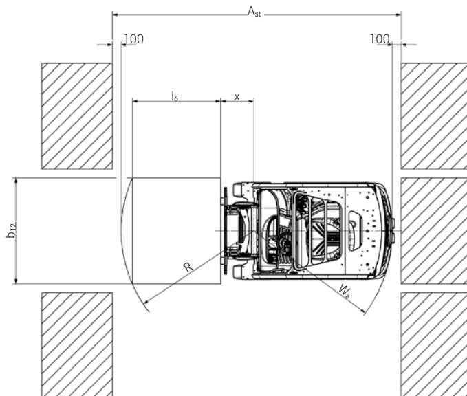
Bovenaanzicht 3 wielen
